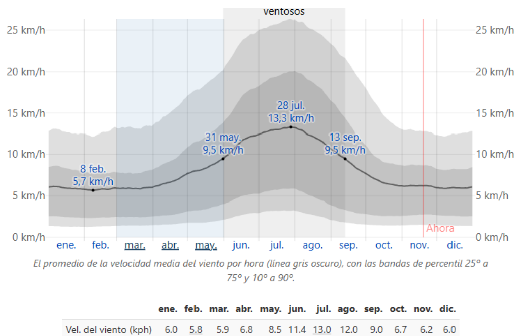
Gráfico 5. Velocidad promedio del viento en Loja
